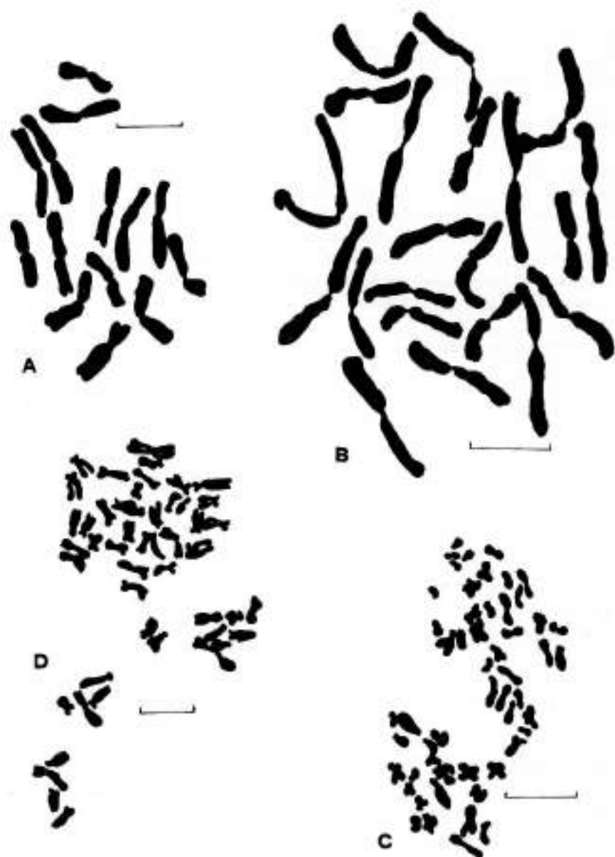
Fig. 3. Karyograms of: A , Allium subhirsutum , 2n = 14 ; B , A. trifoliatum , 2n = 21 ; C , Caruelia arabica , 2n = 50 ; D , Iris sicula , 2n = 48 . — Scale bars = 10 \mu m.
