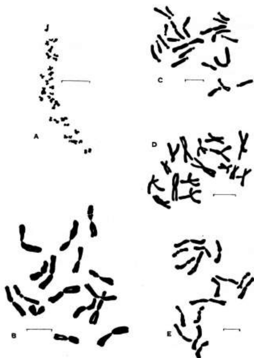
Fig. 2. Karyotypes of: A, Tarasacum minimum , 2n = 32 ; B, Allium arvense , 2n = 16 ; C, A. chamaemoly L. subsp. chamaemoly , 2n = 22 ; D, A. conmutatum , 2n = 16 ; E, A. sphaerocephalon , 2n = 16 . — Scale bars = 10\ \mu\text{m} .
