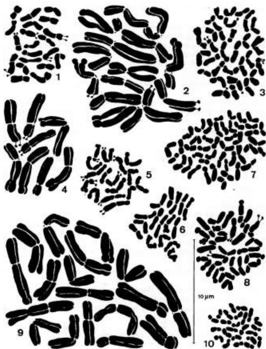
Figs. 1-10. Métaphases somatiques de l'ovaire (Figs. 1 & 5 à 9), méristèmes racinaires (Figs. 2, 3, 10) et mitose pollinique (Fig. 4) de: 1, Legousia speculum-veneris , 2n = 20 ; 2, Lathyrus hirsutus , 2n = 14 ; 3, Ononis minutissima , 2n = 30 ; 4, Ranunculus monspeliacus , n = 8 ; 5, Hypecoum procumbens , 2n = 16 ; 6, Hypecoum torulosum , 2n = 16 ; 7, Galium tricarnutum , 2n = 44 ; 8, Linaria pelixeriana , 2n = 24 ; 9, Melampyrum arvense , 2n = 18 ; 10, Piptatherum miliaceum , 2n = 24 .
